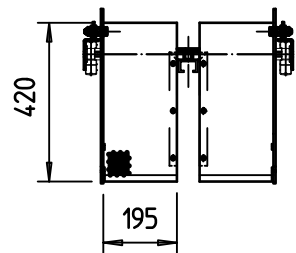
BOVENAANZICHT OPKLAPBAAR WERKBORDES
