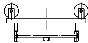
BOVENAANZICHT GEVELWIELSTEL
